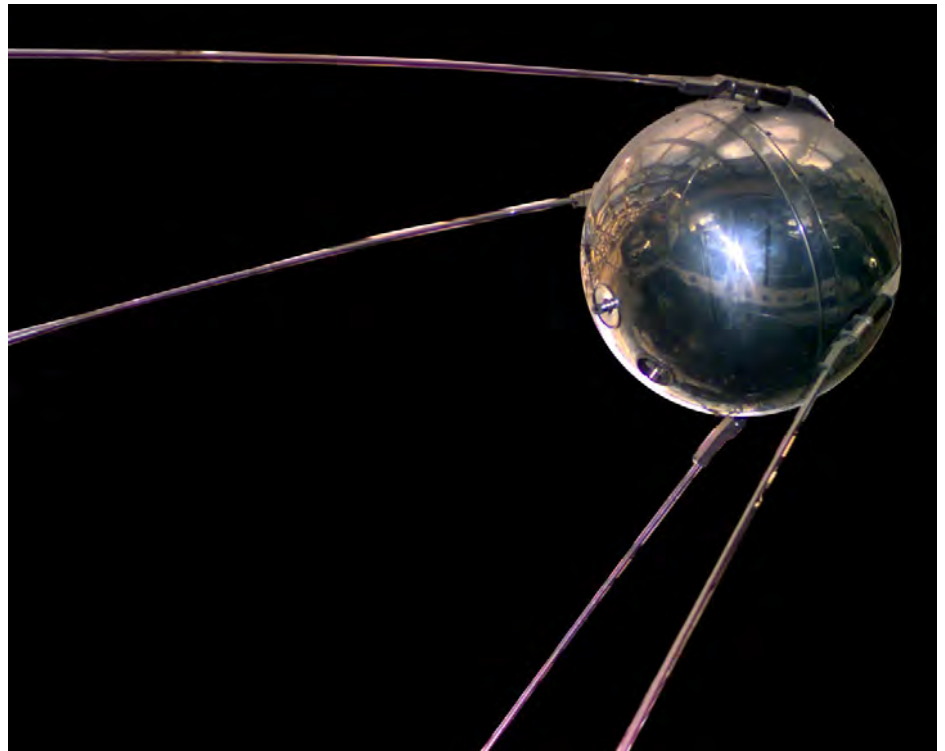
L'Sputnik 1 fou el primer satèl·lit artificial llançat a l'espai. WIKIMEDIA COMMONS
